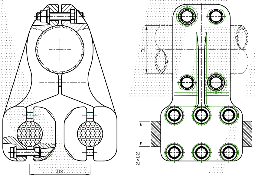
(Tube/wire) to two wires
