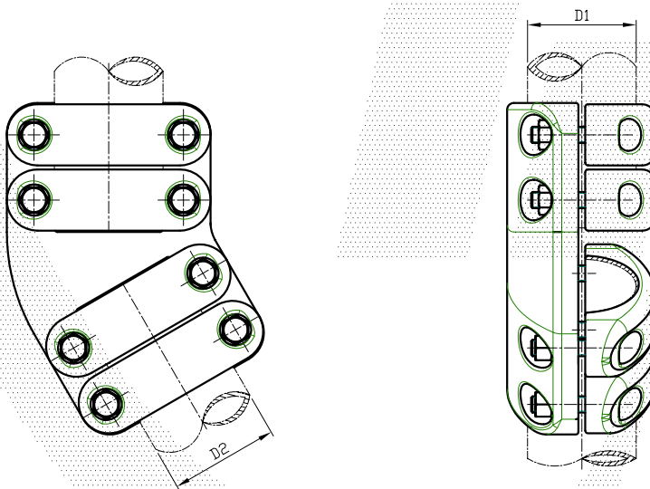
Angle coupler (tube to tube)
